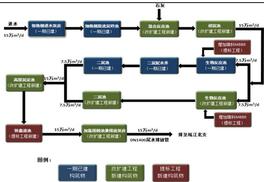
图 4-2 污水处理工艺流程示意图
