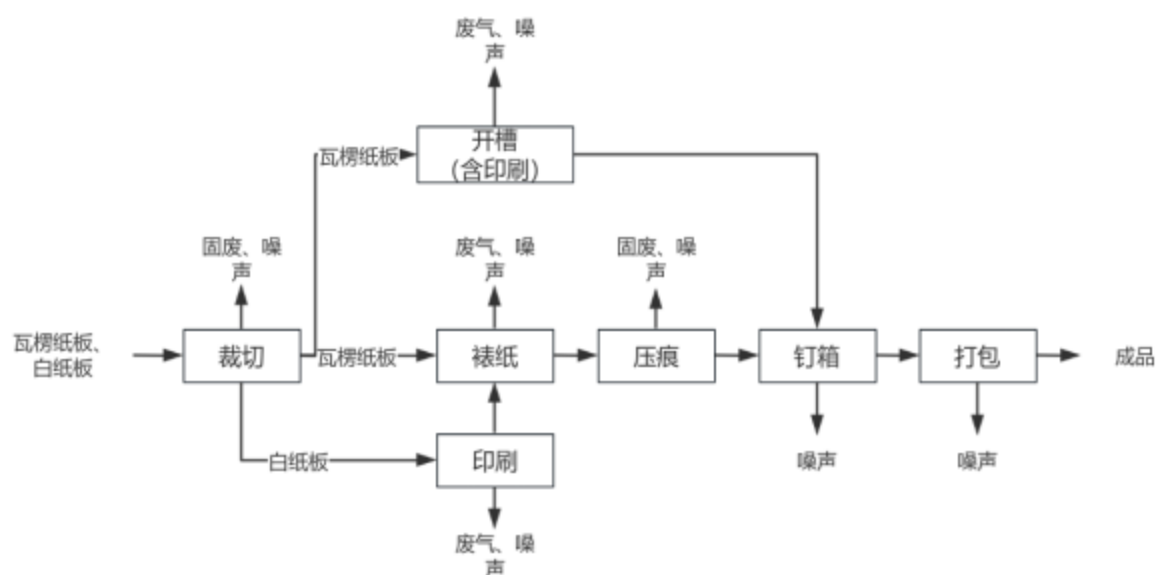
图 2-1 项目生产工艺流程及产污环节示意图
