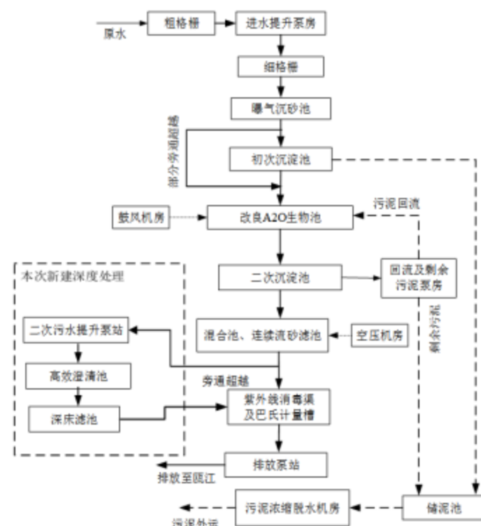
图 4-2 污水处理工艺流程示意图
