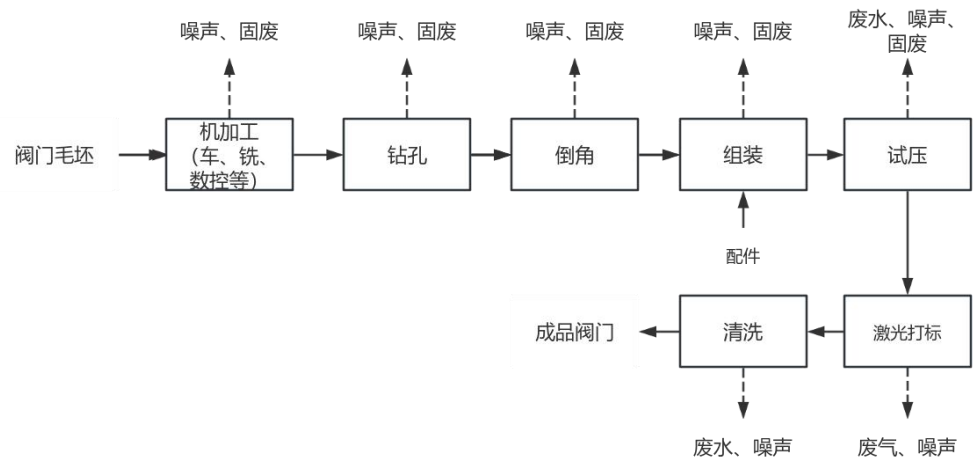
图 2-2 生产工艺流程及产污环节示意图
