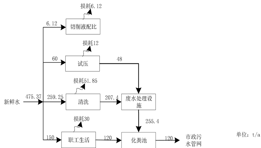
图 2-1 企业水平衡图
