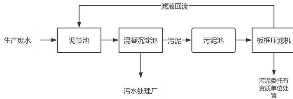
图 4-1 项目生产废水处理工艺流程示意图
