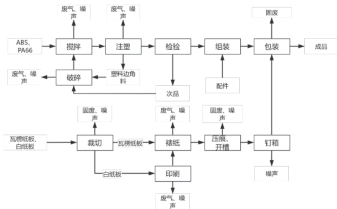
图 2-2 项目塑料开关面板生产工艺流程及产污环节示意图
