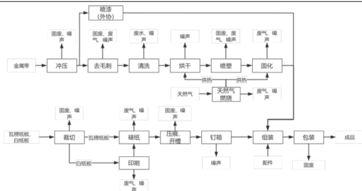
图2-2 项目金属开关面板生产工艺流程及产污环节示意图
