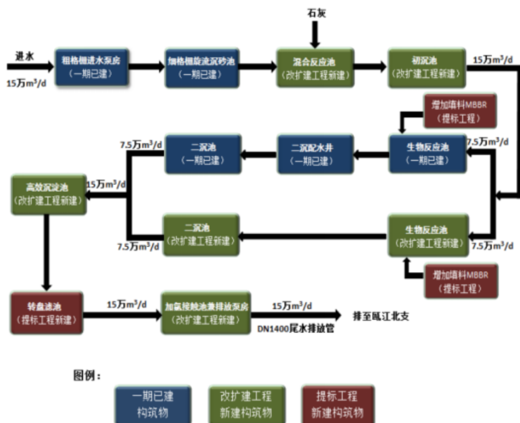
图 4-1 水处理工艺流程示意图
