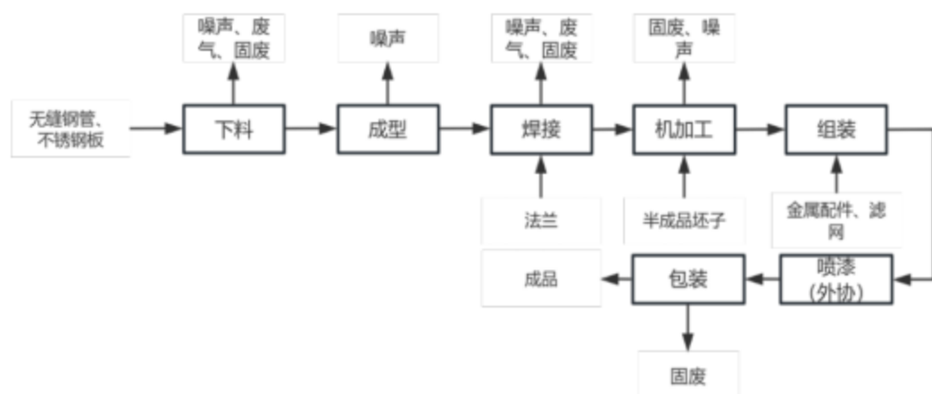
图 2-3 原有项目生产工艺流程及产污环节示意图
