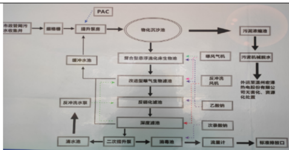
图 4-2 水处理工艺流程示意图
