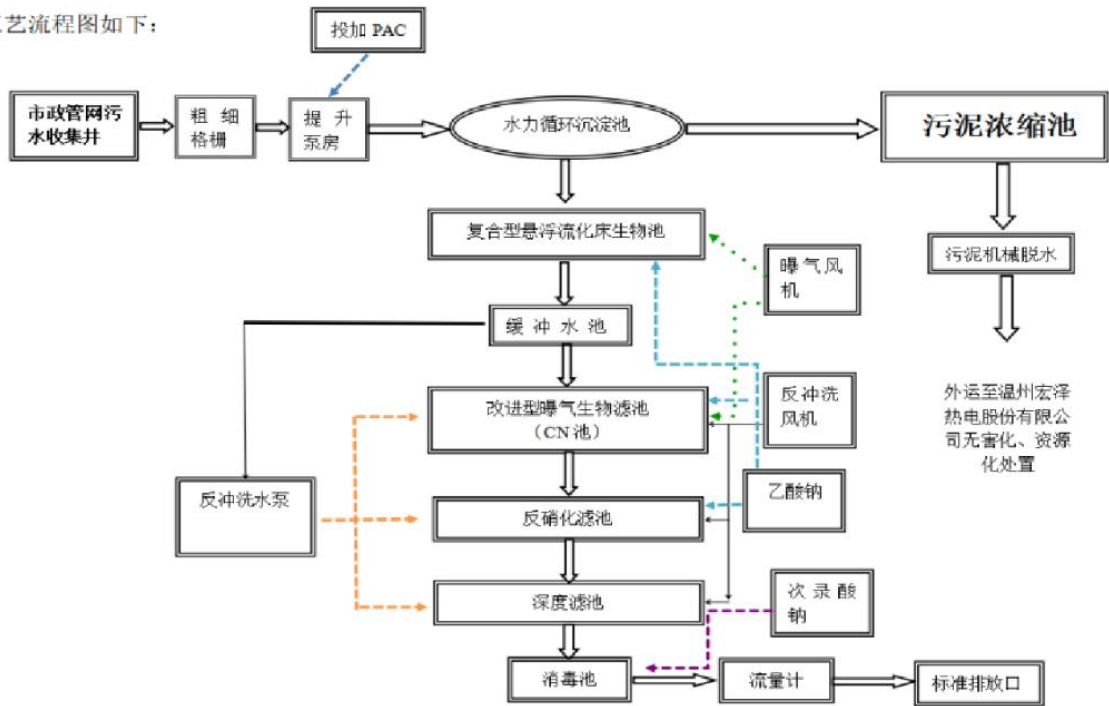
图 4-1 水处理工艺流程示意图
