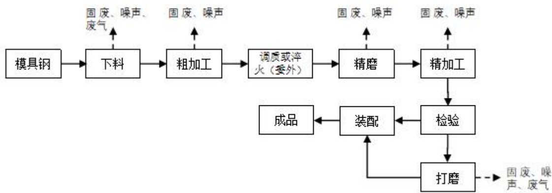
图 2-2 项目生产工艺流程及产污环节示意图
