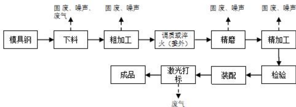
图 2-3 现有项目生产工艺流程及产污环节示意图
