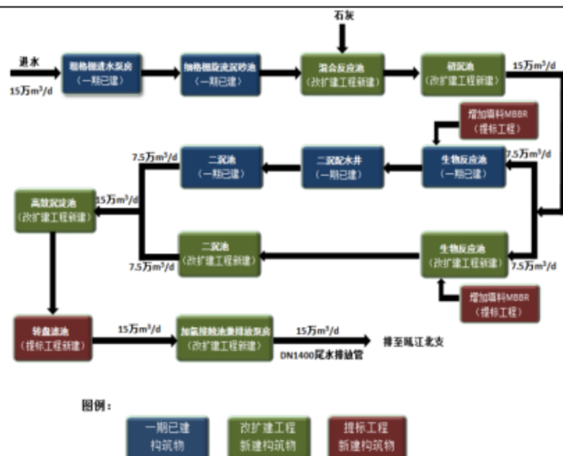
图 4-2 水处理工艺流程示意图
