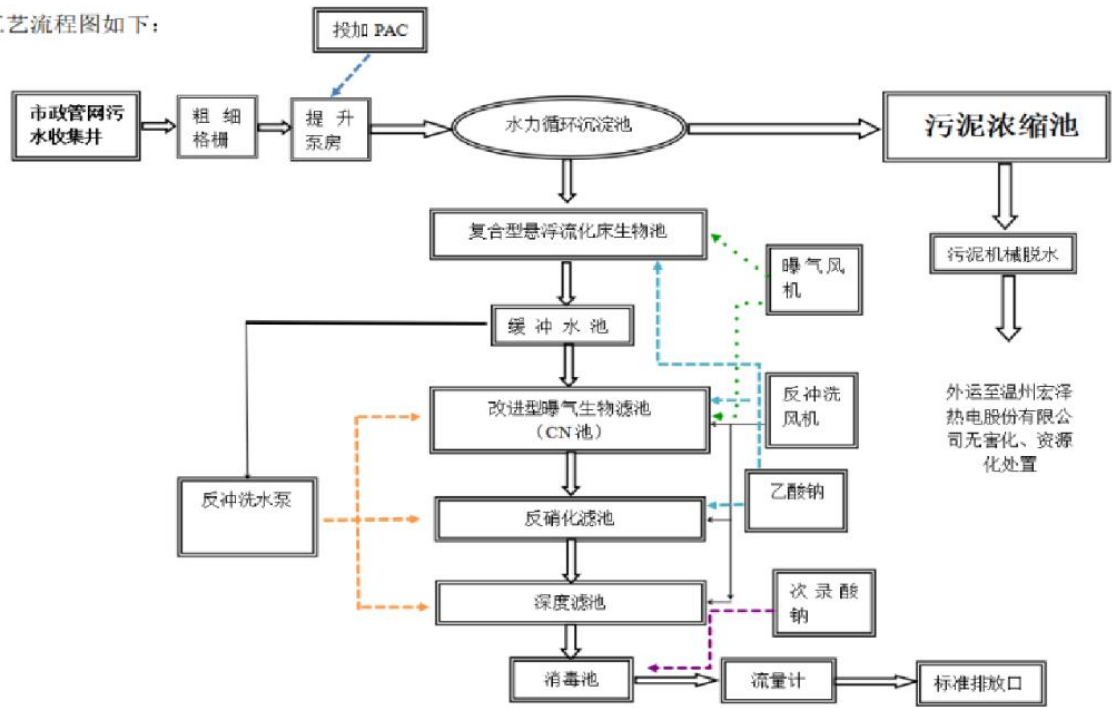
图 4-1 污水处理工艺流程示意图
