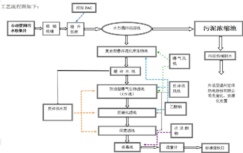
图 4-1 水处理工艺流程示意图
