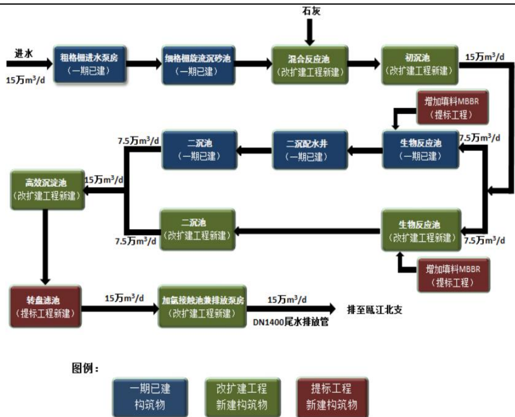
图 4-2 水处理工艺流程示意图
