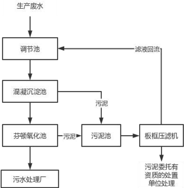
图 4-1 项目生产废水处理工艺流程示意图
