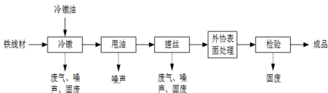
图 2-1 项目运营期工艺流程及产污环节示意图
