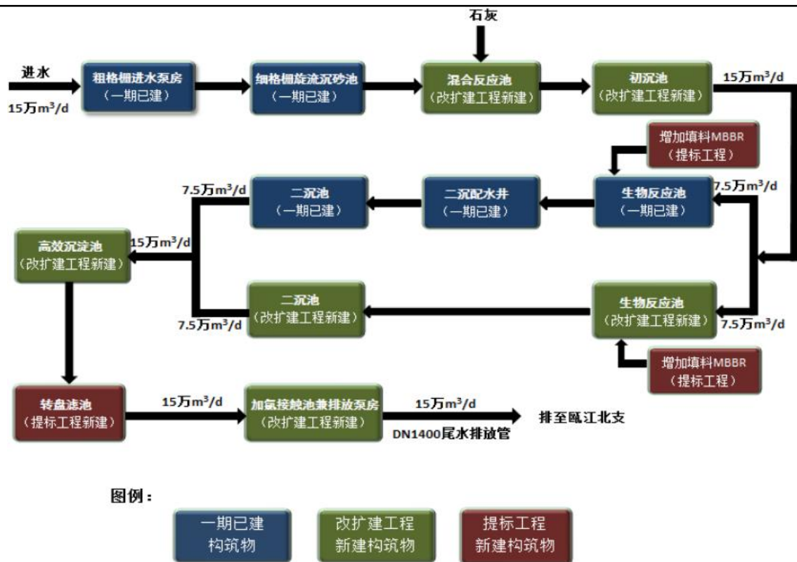
图 4-2 水处理工艺流程示意图
