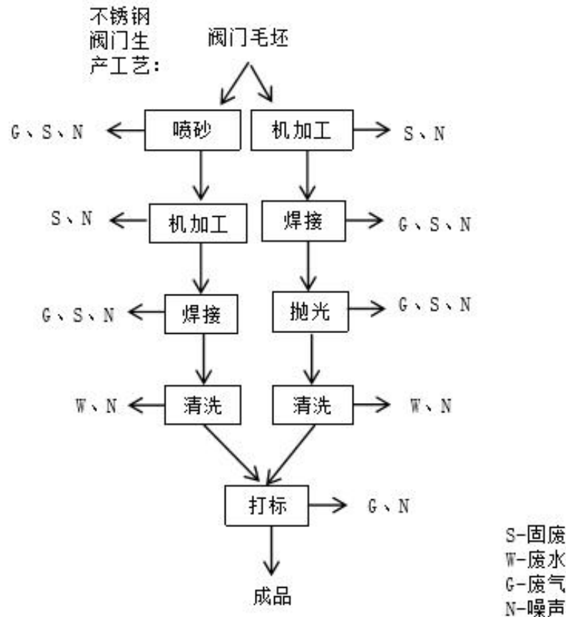
图 2-2 项目不锈钢阀门生产工艺流程及产污环节示意图
