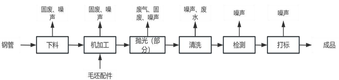
图 2-2 项目生产工艺流程及产污环节示意图
