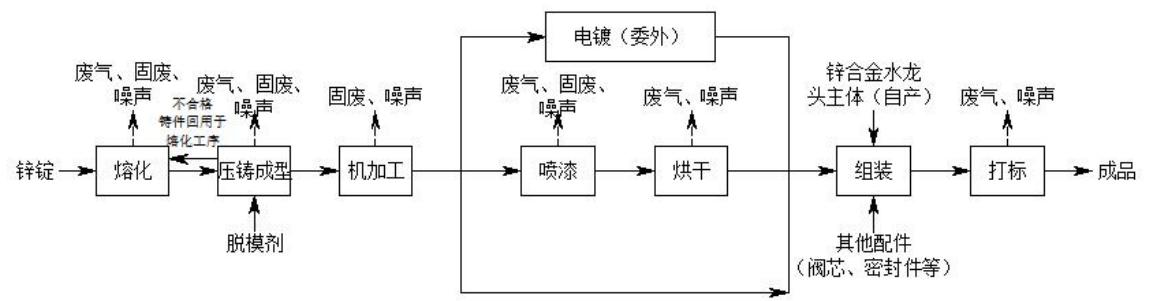
图 2-3 项目锌合金水龙头生产工艺流程及产污环节示意图
