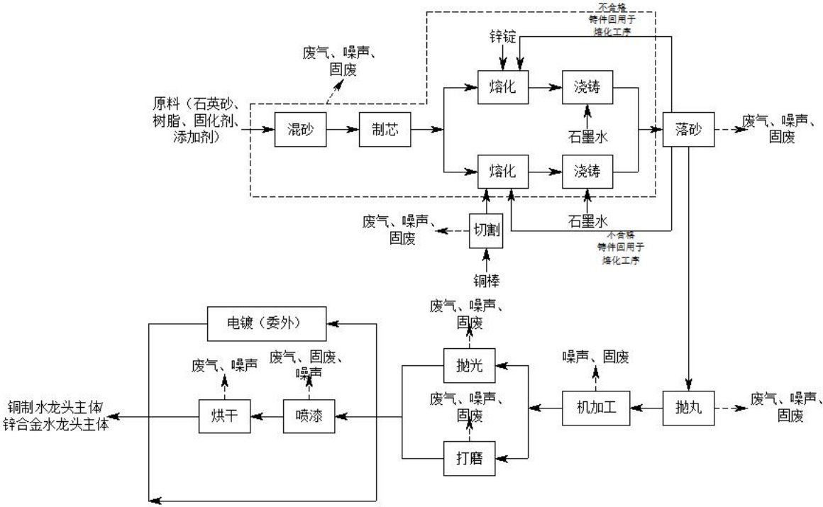
图 2-2 项目水龙头主体（铜合金、锌合金）生产工艺流程及产污环节示意图
