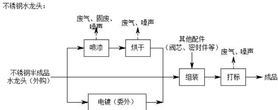
图 2-5 项目不锈钢水龙头生产工艺流程及产污环节示意图
