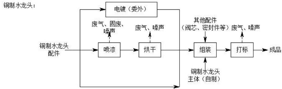
图 2-4 项目铜制水龙头生产工艺流程及产污环节示意图
