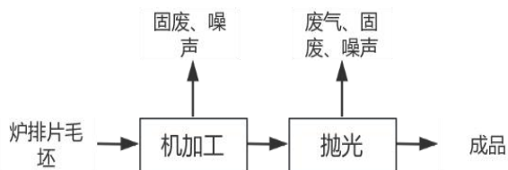
图 2-3 项目炉排片生产工艺流程及产污环节示意图
