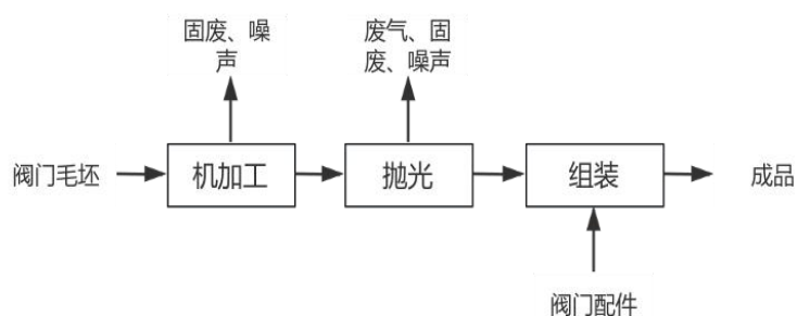
图 2-2 项目阀门生产工艺流程及产污环节示意图
