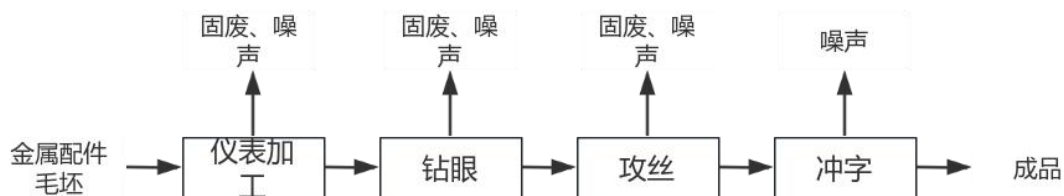
图 2-4 项目金属配件生产工艺流程及产污环节示意图
