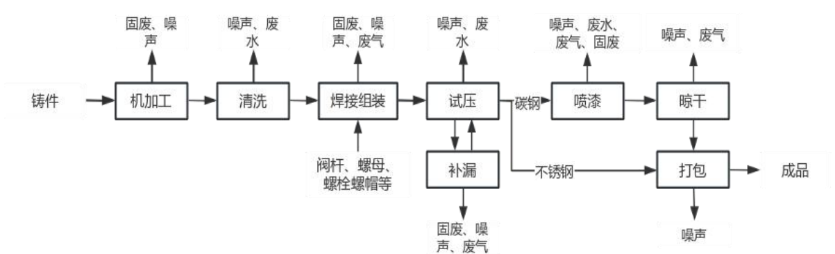
图 2-2 阀门生产工艺流程及产污环节示意图
