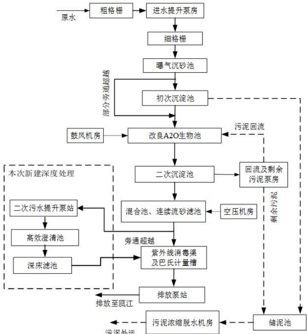
图 4-2 污水处理工艺流程示意图
