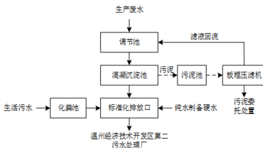
图 4-1 项目废水处理工艺流程示意图
