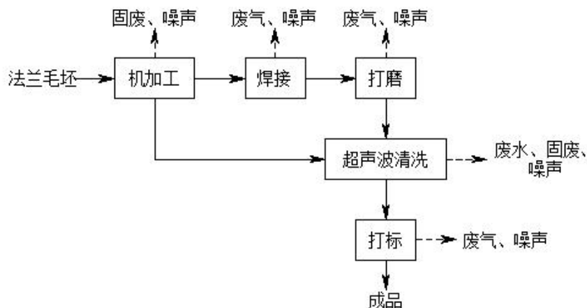
图 2-2 项目法兰生产工艺流程及产污环节示意图
