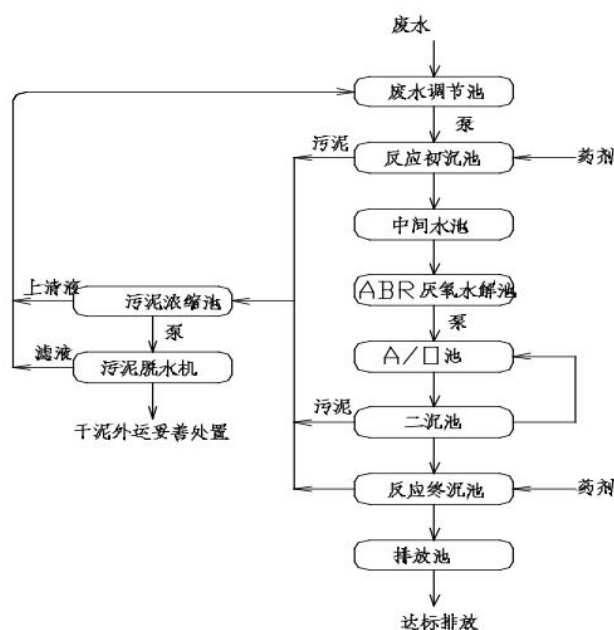
图 4-2 水处理工艺流程示意图
