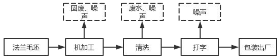
图 2-2 生产工艺流程及产污环节示意图
