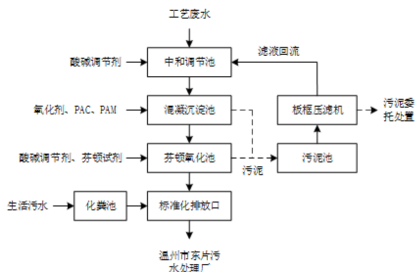
图 4-1 项目废水处理工艺流程示意图
