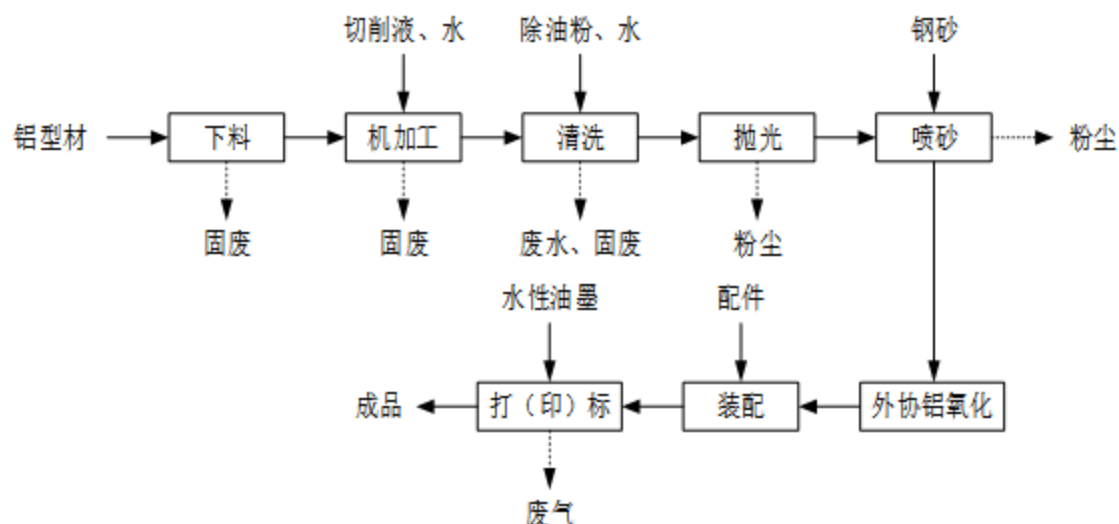
图 2-2 项目工艺流程及产污环节示意图
