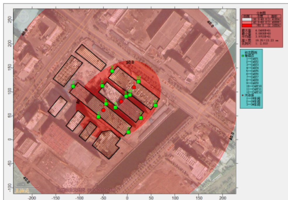
图 4-4 项目厂界噪声预测结果图
