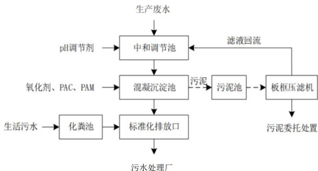
图 4-1 项目生产废水处理工艺流程示意图
