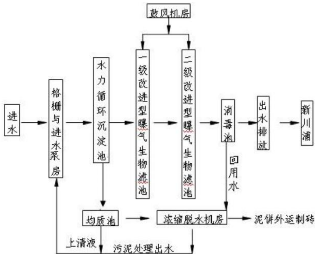
图 4-2 污水处理工艺流程示意图
