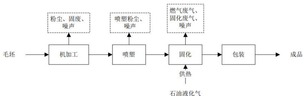
图 2-3 原有项目生产工艺流程及产污节点图
