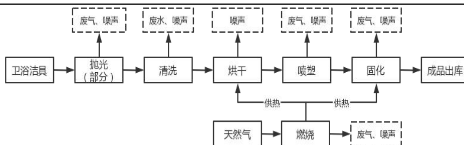
图 2-2 项目生产工艺流程及产污环节示意图
