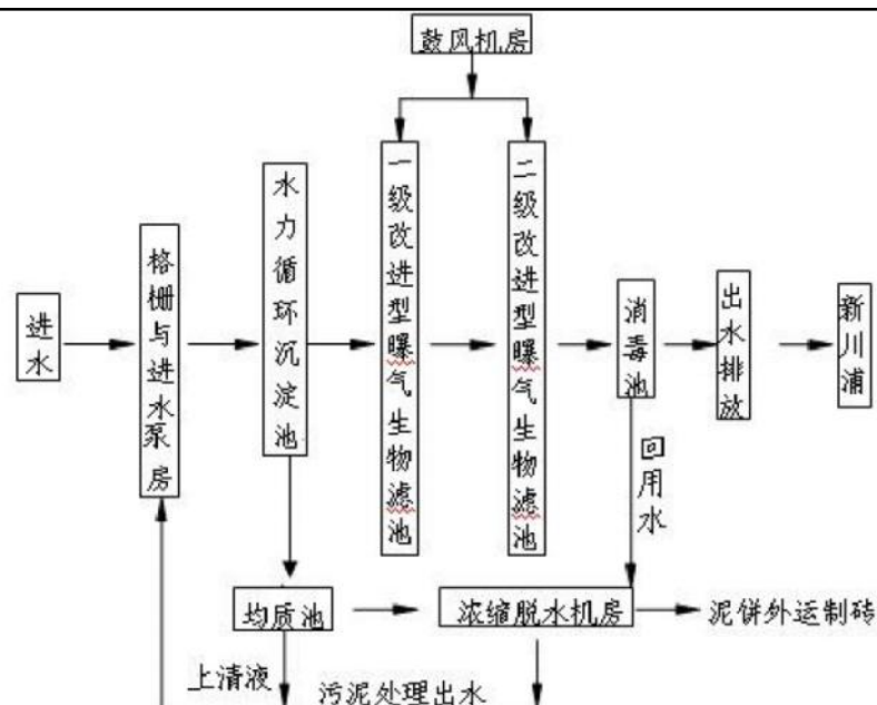
图 4-1 污水处理工艺流程示意图
