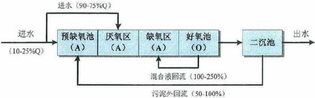
图 4-1 水处理工艺流程示意图
