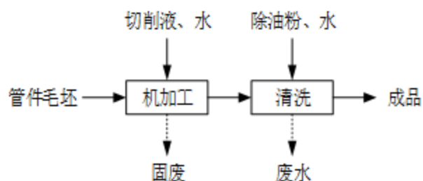
图 2-3 项目管件生产工艺流程及产污环节示意图
