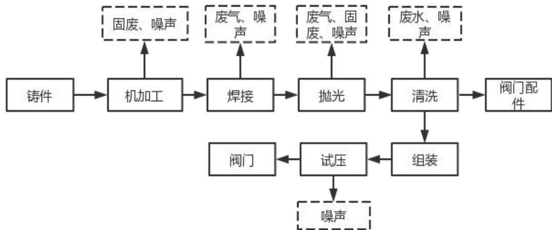
图 2-2 阀门、阀门配件生产工艺流程及产污环节示意图
