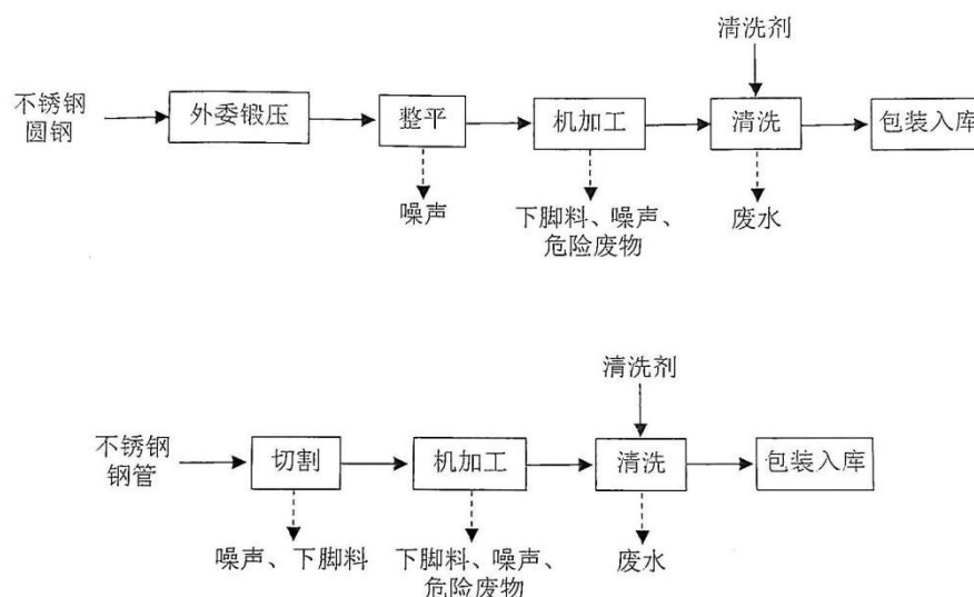
图 2-5 原有项目阀门管件生产工艺流程及产污环节示意图
