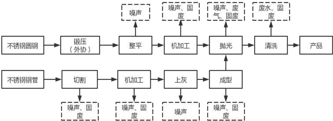
图 2-3 阀门管件生产工艺流程及产污环节示意图
