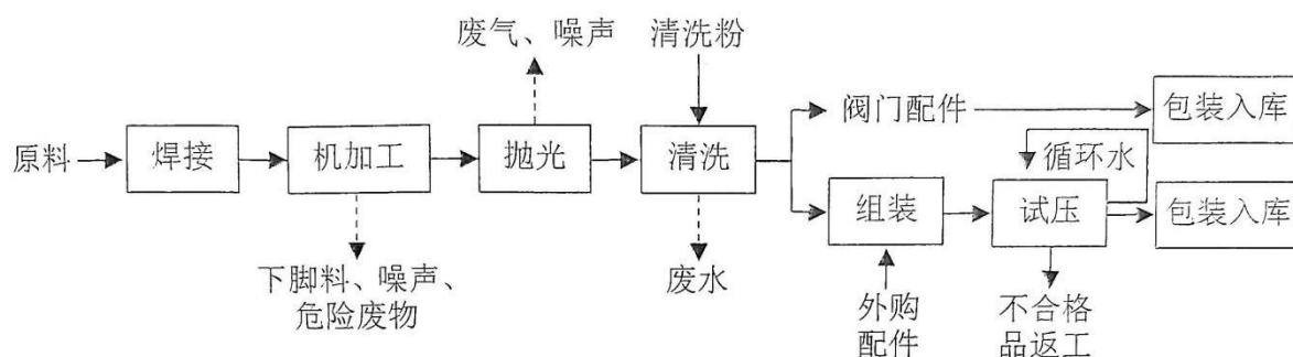
图 2-4 原有项目阀门、阀门配件生产工艺流程及产污环节示意图
