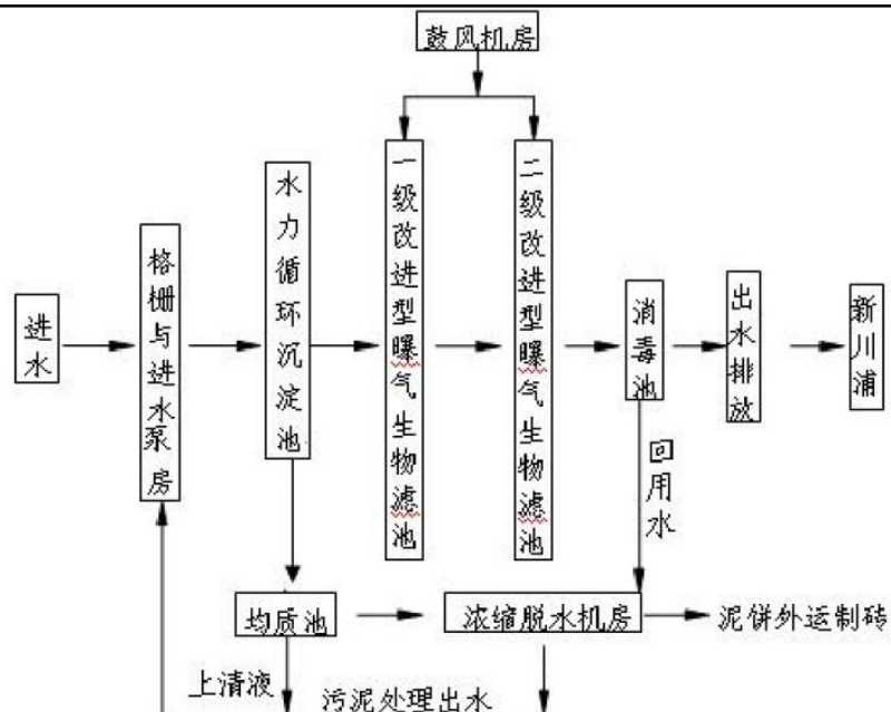
图 4-1 污水处理工艺流程示意图
