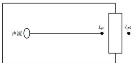
图 4-3 室内声源等效为室外声源示意图
