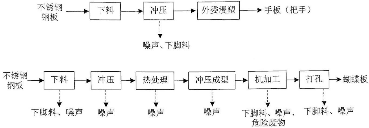
图 2-6 原有项目蝴蝶板、手板（把手）生产工艺流程及产污环节示意图
