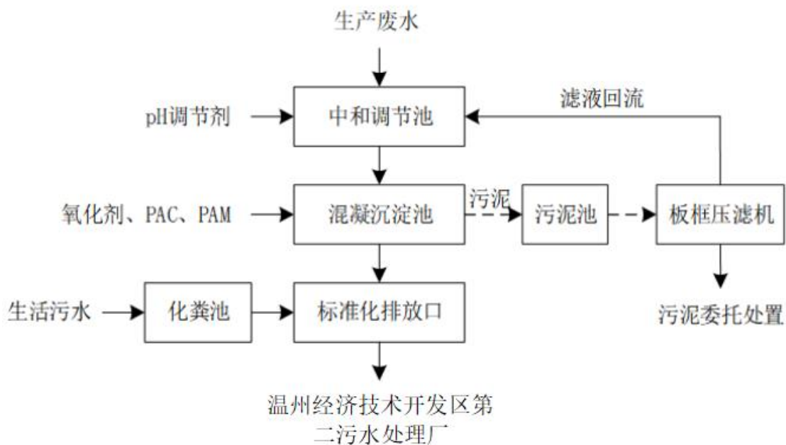
图 4-1 项目生产废水处理工艺流程示意图
