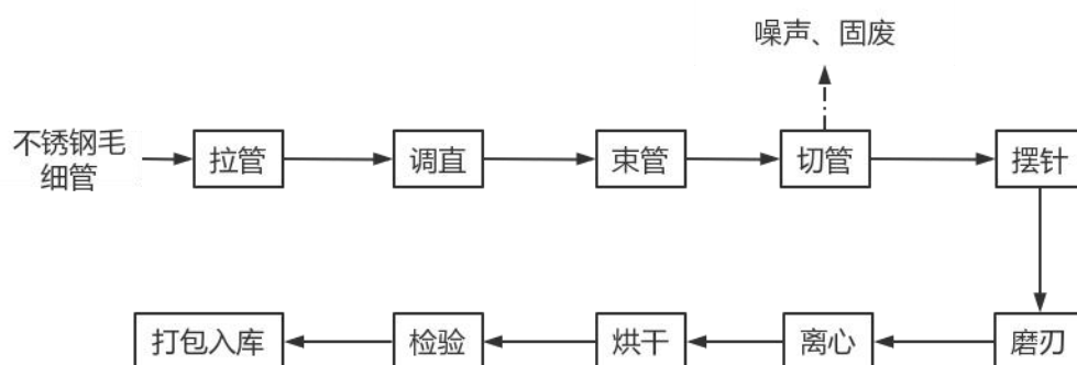
图 2-2 生产工艺流程及产污环节示意图
